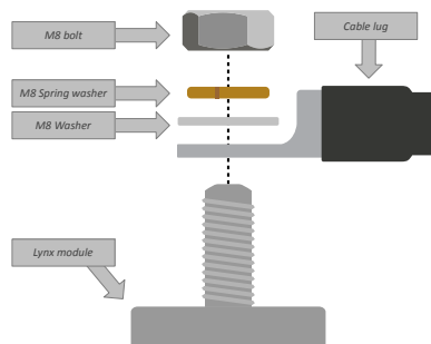
Abbildung 3. Richtige Montagesequenz der Gleichstromleitungen
