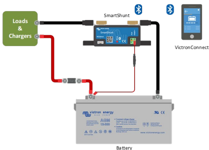
Grundlegende SmartShunt-Verkabelung
